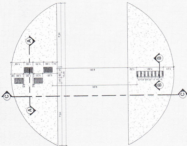
01 PLANTA BAIXA 1:100
