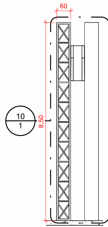
02 CORTE AA 1 : 100
