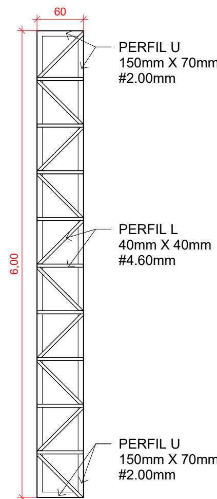
09 Pilar 6,00 1 : 50
