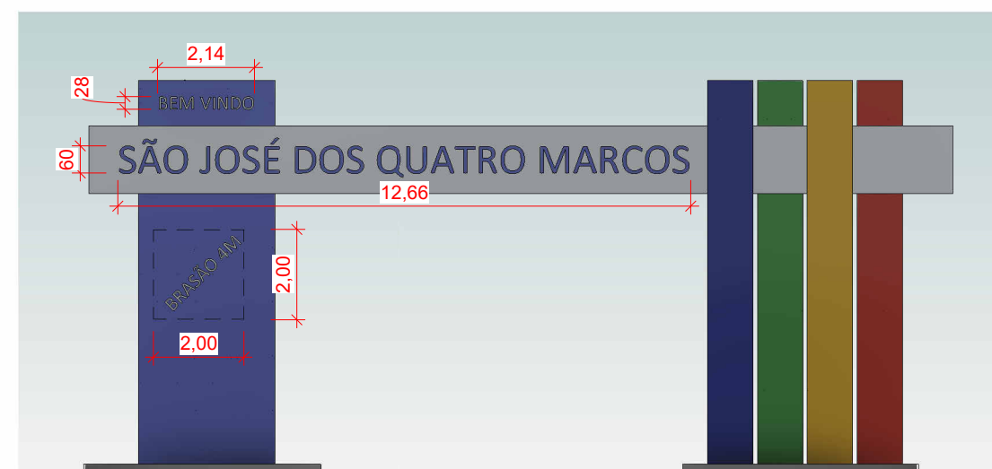
05 FACHADA LESTE 1 : 150
