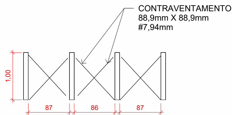
07 Contraventamentos 1,37 1 : 50
