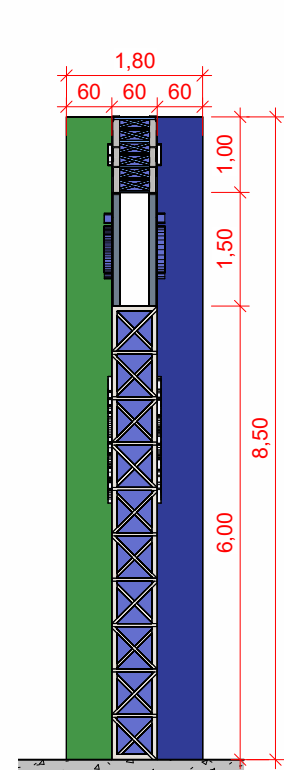
05 CORTE BB 1 : 100
