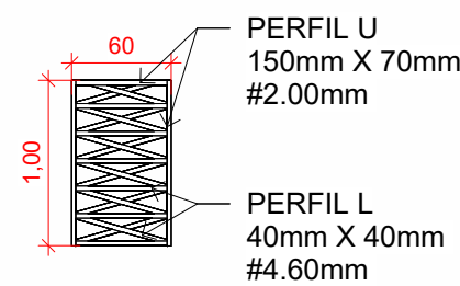
08 Pilar 1,00 1 : 50
