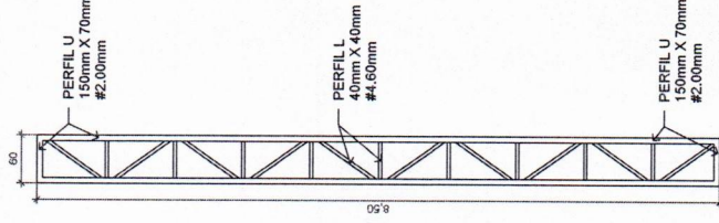
10 Pilar 8.50 1:50
