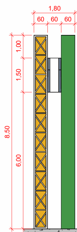
06 CORTE AA 1 : 100
