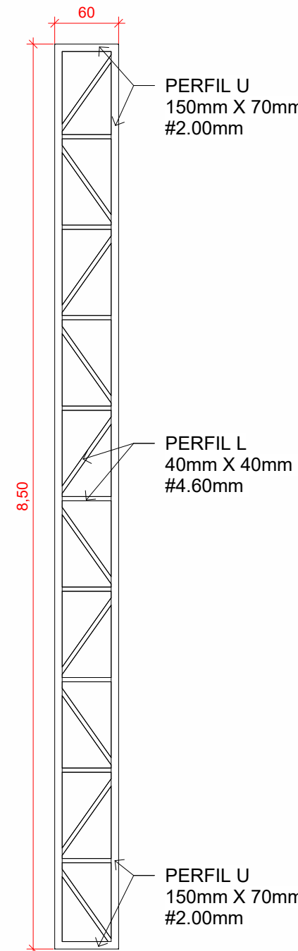
10 Pilar 8,50 1 : 50
