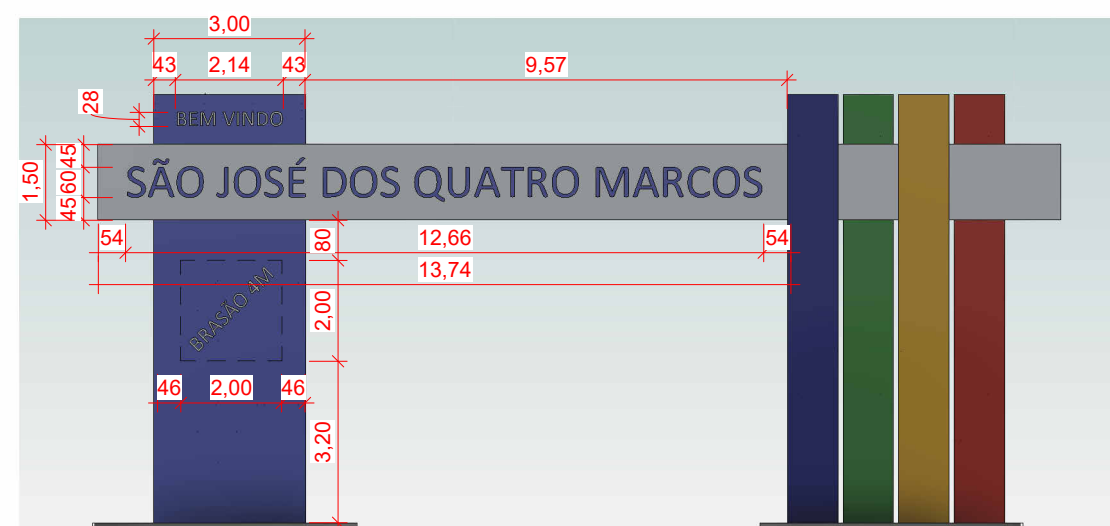
04 FACHADA LESTE - ARQ 1 : 150
