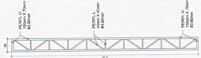
10 Pilar 8,50 1:50
