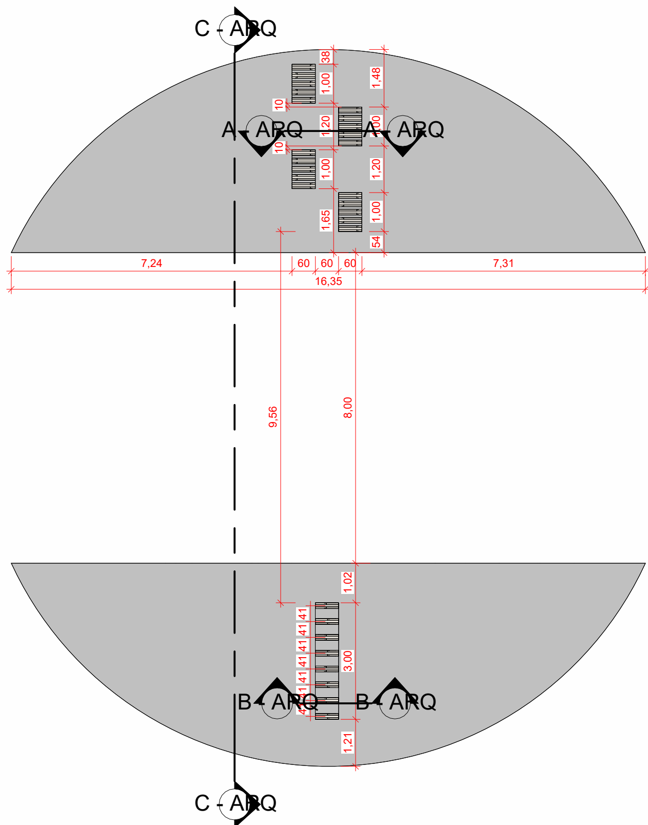
01 PLANTA BAIXA - ARQ 1 : 100
