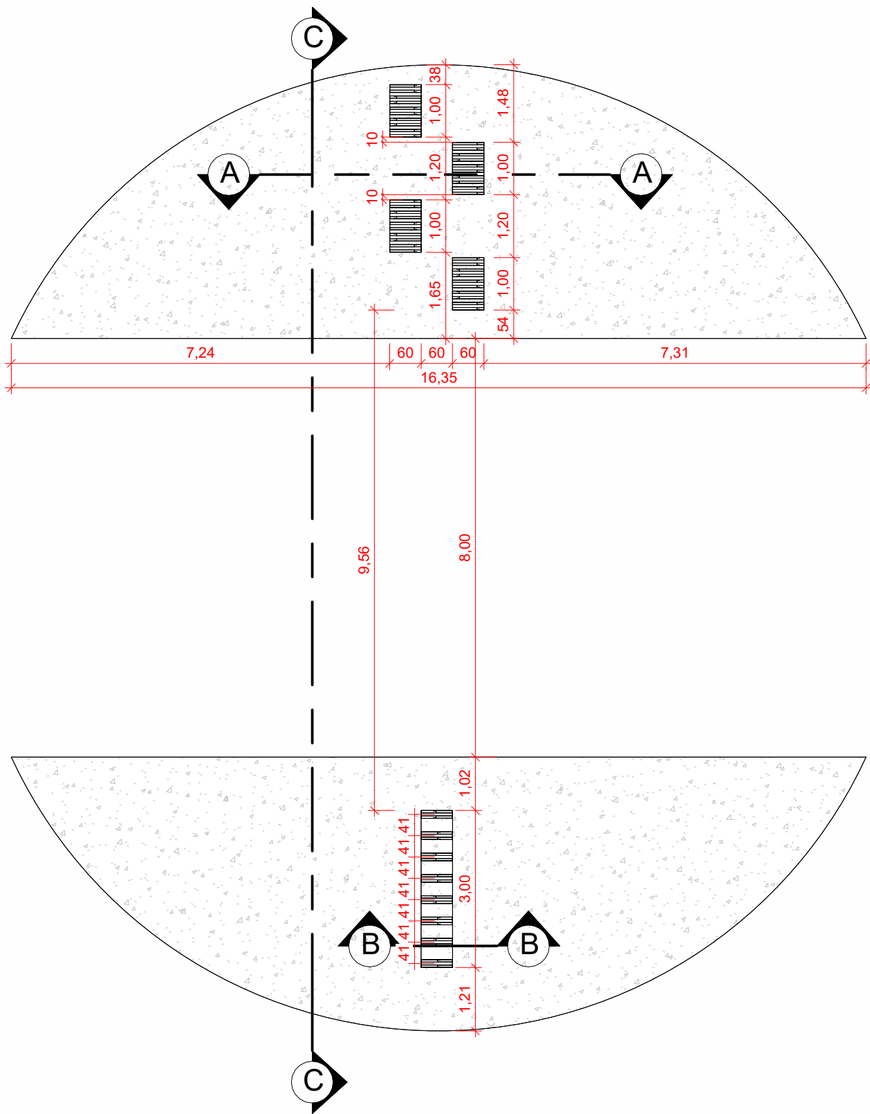
01 PLANTA BAIXA 1 : 100
