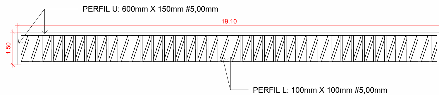
06 Viga 19,10 1 : 100
