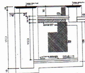
FILTRO ANAERÓBIO CORTE - ESC. 1:25
