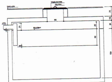
TANQUE SÉPTICO CORTE - ESC. 1:25
