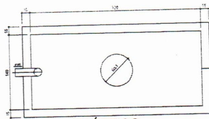
TANQUE SÉPTICO PLANTA BAIXA - ESC. 1:25
