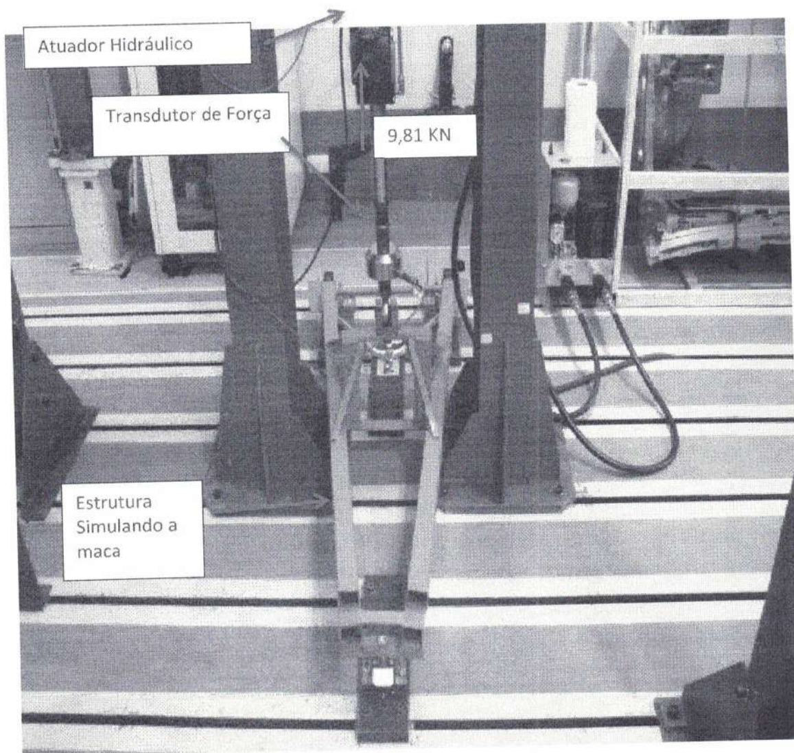
Figura 11 – Bancada de teste para ensaio vertical.
